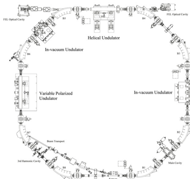
Fig. 1 UVSOR-II電子蓄積リング (2006年10月現在)
