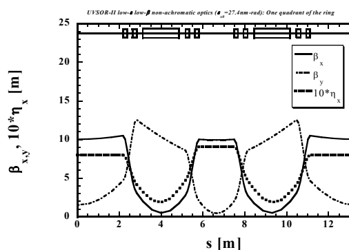
Fig. 2 UVSOR-IIのビームオプティクス
