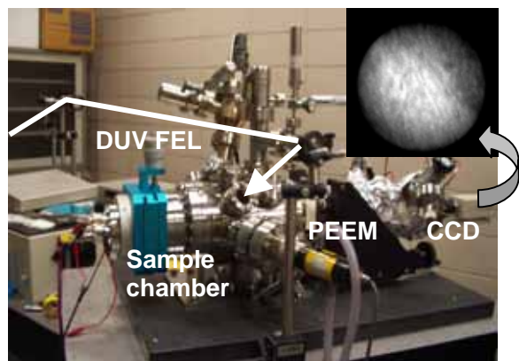
図5 : FEL-PEEMシステム
