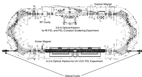
図1: NIJI-IV FELシステム
