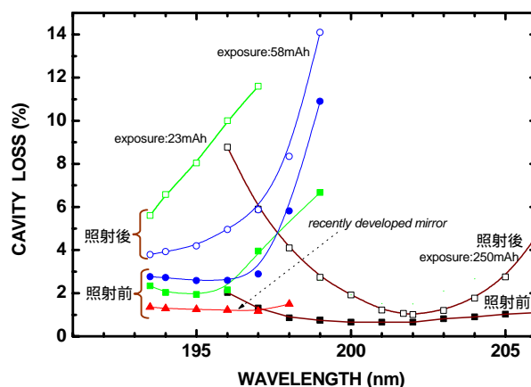
図2: 共振器損失の波長依存性
