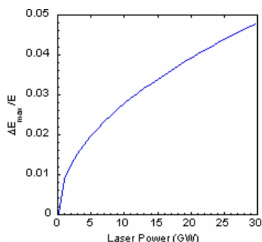
図2 modulator内でのレーザーピークパワーに対する電子ビームのエネルギー変調。適切なレーザー集束条件を仮定した。
