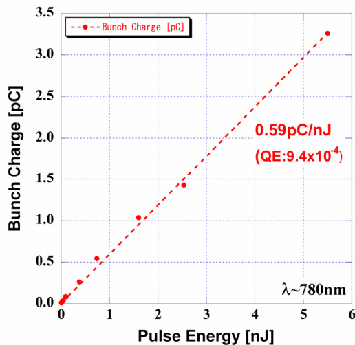
図4：パルス幅 25ps のレーザ光を照射した時の GaAs/GaAsP 超格子フォトカソードからのビーム引出し結果。
