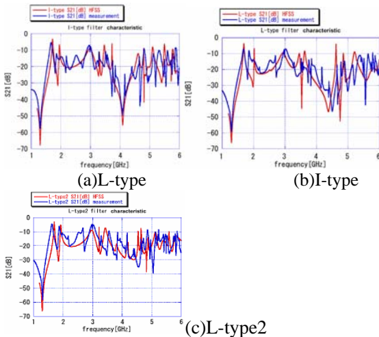
図3 HOMカップラの周波数特性の比較
