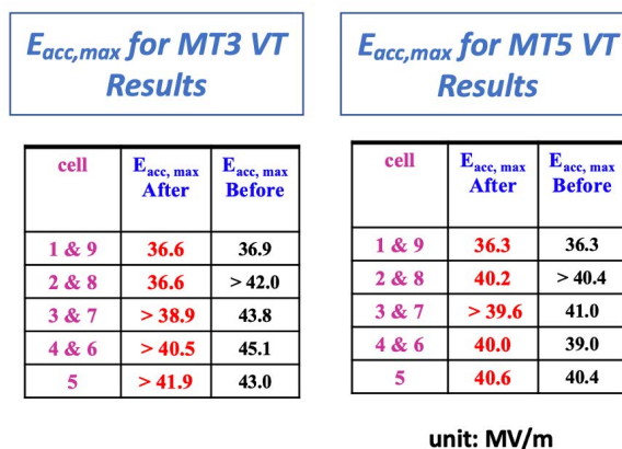
Figure 8: 2-step baking 前後の電界性能の変遷。
