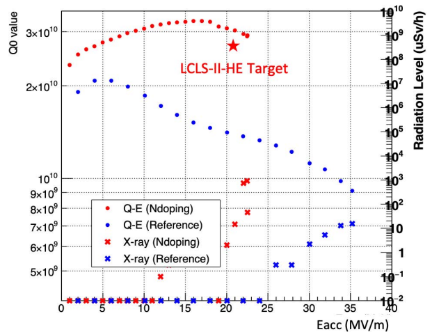
Figure 11: N-doping 空洞の電界性能の評価。
